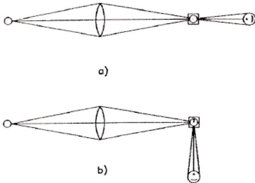
Figura 1: a) schema di torbidimetro; b) schema di nefelometro.
